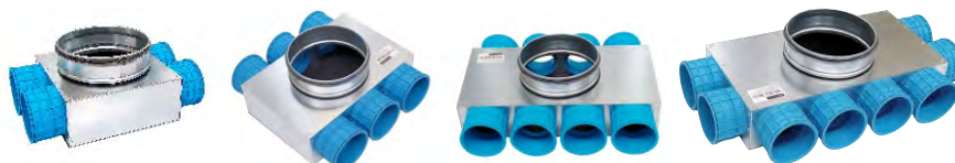
IPRKJX Ø160 / 4x Ø75 (0202) IPRKJX Ø160 / 6x Ø75 (0303) IPRKJX Ø160 / 8x Ø75 (0404) IPRKJS Ø160 / 8x Ø75 (2420)
